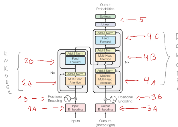
Rysunek 11: Obrazek przedstawia schemat działania transformera z opisami potrzebnymi do dalszego opisu.
